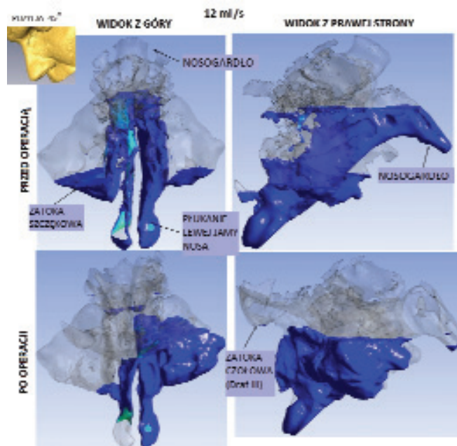
Ryc. 3. Porównanie płukania zatok przynosowych przed operacją i po operacji. Źródło: Zhao K. i in., Sinus irrigations before and after surgery – visualization through computational fluid dynamics simulations . Laryngoscope , 2016, 126(3), s. 90-96.
